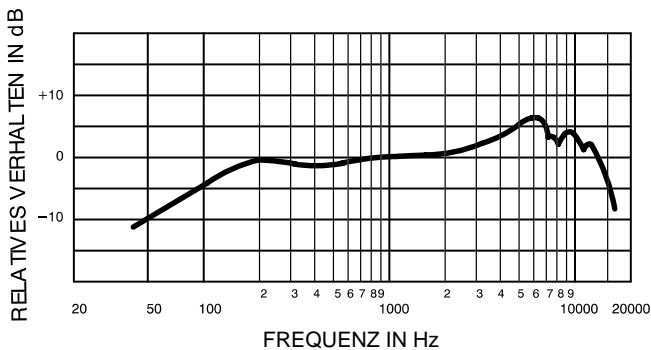
TYPISCHES FREQUENZGANG ABBILDUNG 2
