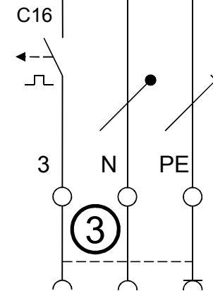
3 x Schuko
