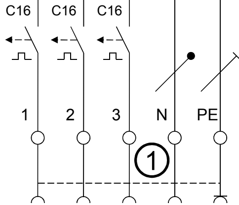
2 x CEE 16 A
