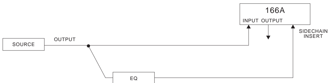
Abb. 3: Frequenzselektive Kompression
